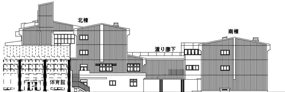
西立面図
