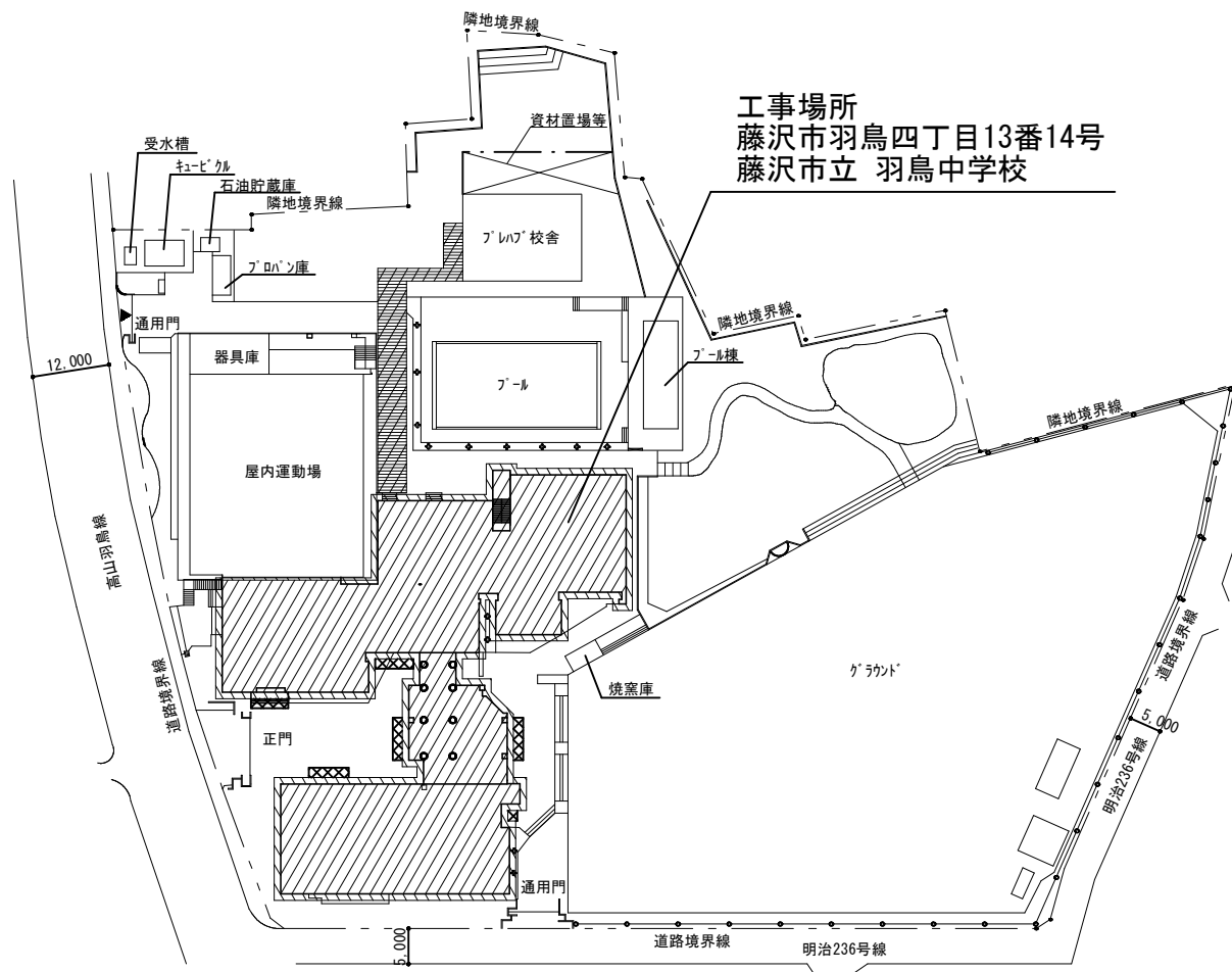
配置図
