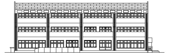
南棟 南立面図
